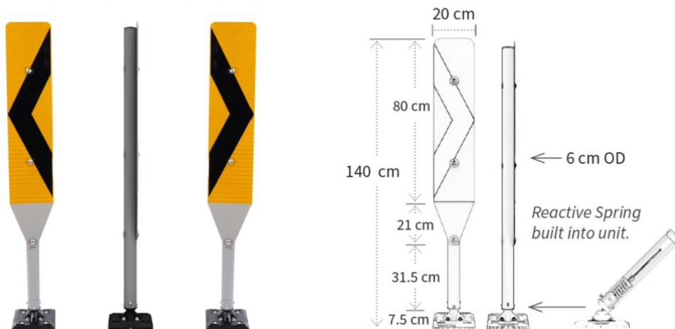
Vooraanzicht Zij aanzicht Vooraanzicht
